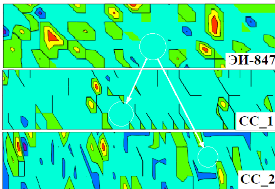
Рисунок 7 – Сравнение потенциграмм, построенных для CC_1 и CC_2, а также для образца из стали ЭИ-847, деформированного при растяжении (результаты приведены для значения уровня фиксации SLS=3,523) [Comparison of potentiograms constructed for CC_1 and CC_2 as well as for a specimen made of steel EI-847, deformed under tension (the results are given for the value of the fixation level SLS = 3.523)]
