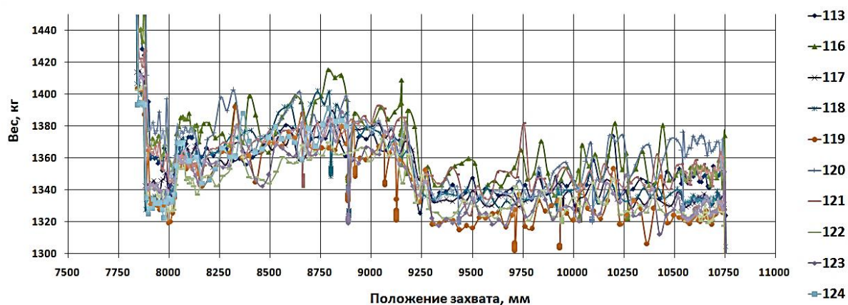
Рисунок 4 – График зависимости весовой нагрузки на ЗРШ от его положения для ТВС, облученных в течение трех кампаний при выгрузке из реактора [The graph of the dependence of the weight load on the working rod gripper on its position for fuel assemblies irradiated during three campaigns during unloading from the reactor]
