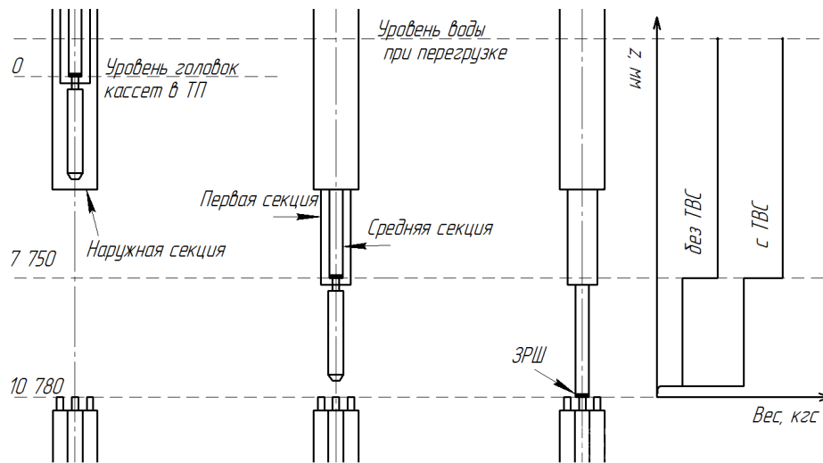
Рисунок 5 – Высотная схема расположения ЗРШ и кассет High-altitude layout of working rod gripper and cassettes]
