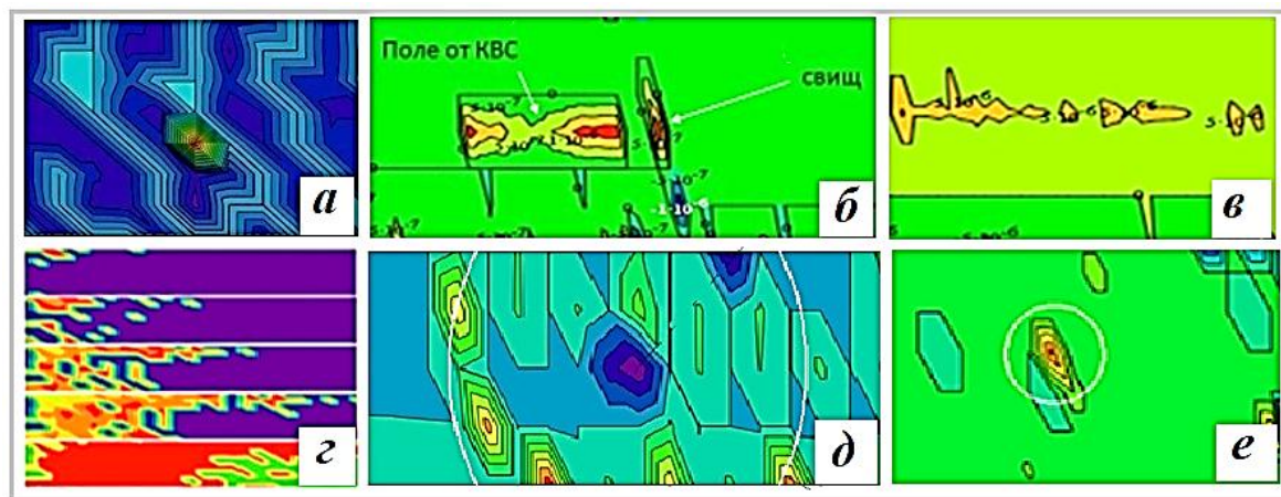
Рисунок 2 – Примеры рефлексов, относящихся к различным структурным неоднородностям в образцах из стали и в сварных соединениях стальных пластин: а – рефлекс области формирования зародыша микроскопической трещины при растяжении стали ЭИ 847 (SLS= 4,699); б – поле упругих напряжений вокруг вольфрамового осколка и рядом расположенный с ним свищ в сварном соединении (SLS= 5,699); в – непровар корня в сварном соединении двух стальных пластин (SLS= 4,301); г – процесс образования мартенсита при растяжении стали 12X18H10T (SLS~5), показанный на пяти отдельных потенциограммах; д – небольшой кусок молибдена (в центре рисунка), помещенный на дно конической воронки в стальном бруске и заваренный там. Видны также рефлексы от линии основания конуса (SLS= 2,155); е – молибденовый цилиндр, помещенный по посадке с зазором в отверстие стальной пластины и заваренный там (SLS= 5,238) [Examples of reflections related to various structural inhomogeneities in steel specimens and in welded joints of steel plates: a – reflex of the area of formation of a microscopic crack nucleus during tension of EI 847 steel (SLS = 4.699); b – the field of elastic stresses around the tungsten fragment and a hole located next to it in the welded joint (SLS = 5.699); c – lack of root penetration in the welded joint of two steel plates (SLS = 4.301); d – the process of formation of martensite during tension of steel 12X18H10T (SLS ~ 5), shown in five separate potentiograms; e – a small piece of molybdenum (in the center of the figure), placed at the bottom of a conical funnel in a steel bar and welded there. Reflexes from the line of the base of the cone are also visible (SLS = 2.155); e – a molybdenum cylinder placed along a gap fit into a hole in a steel plate and welded there (SLS = 5.238)]
