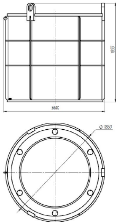
Рисунок 1. Контейнер для хранения выемной части ГЦН.
