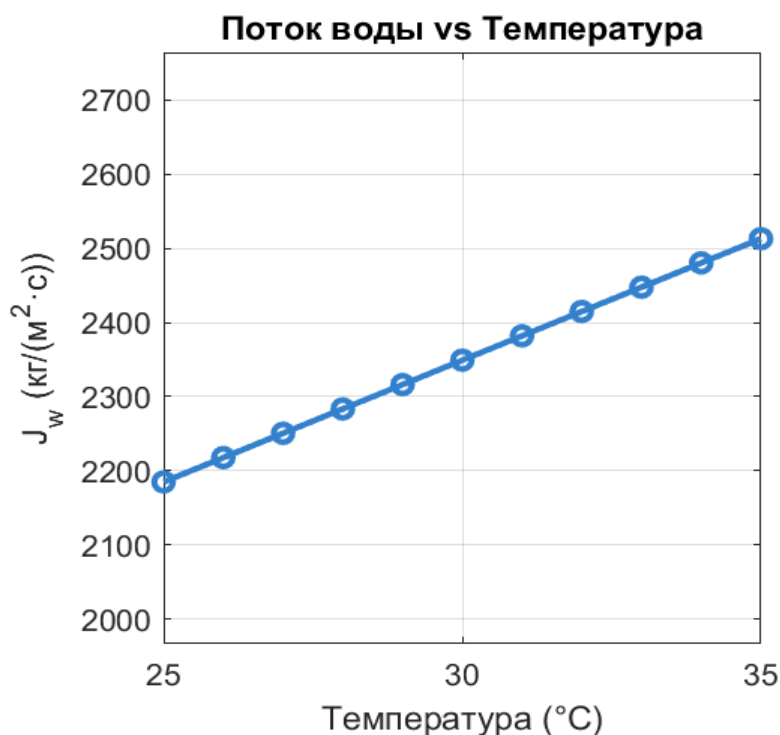
Рисунок 2 - Зависимость удельного потока воды от температуры
