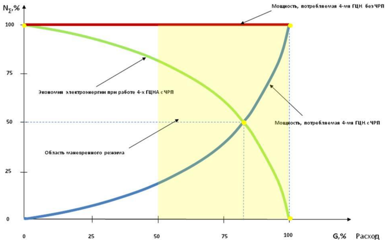
Рисунок 1 - График работы 4-х ГЦНА с ВЧРП и без ВЧРП
