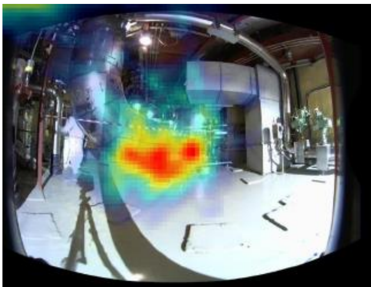
Рисунок 1 – Локализация Ag-110m, место измерения – третья петля ГЦТ
