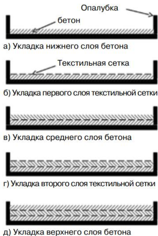
Рисунок 1 - Схема приготовления текстиль-бетона
