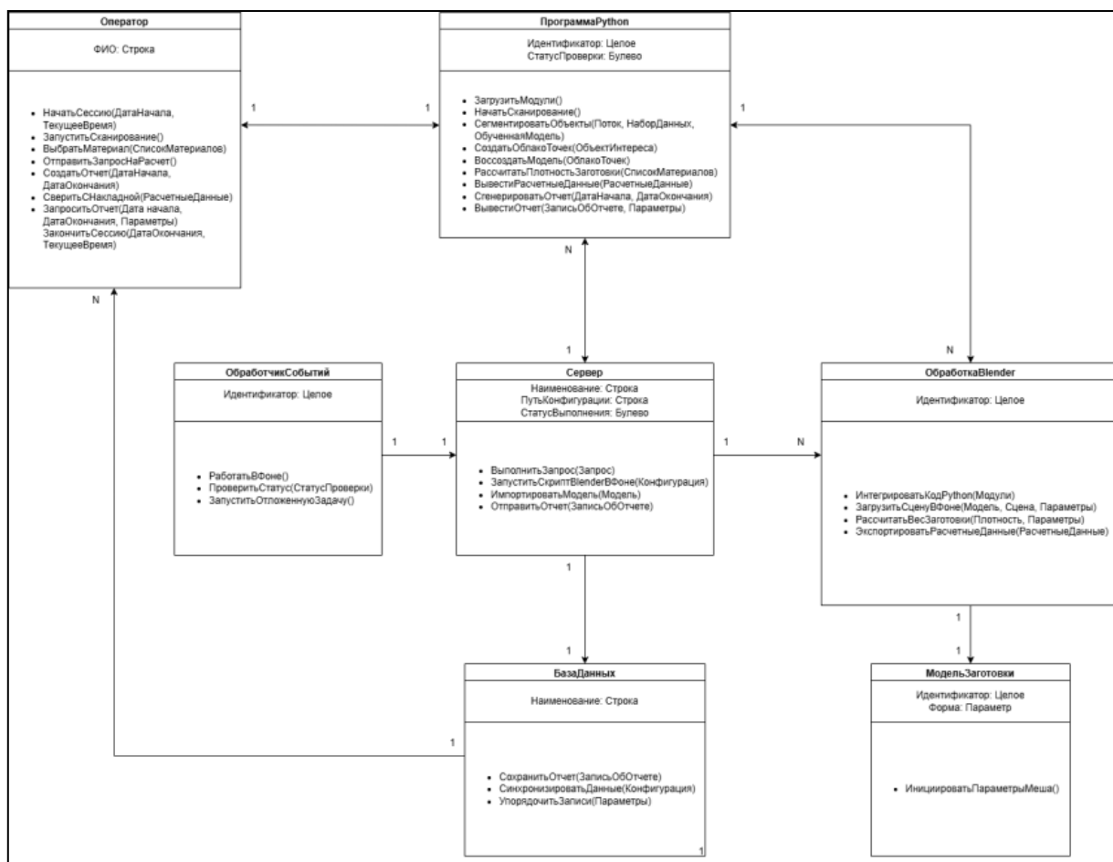
Рисунок 2 – Диаграмма классов
