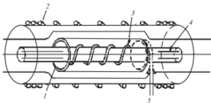
Рисунок 1 – Модернизированный бетатрон. 1 - электронный пучок; 2 – катушка бетатронного поля; 3 – катушка бетатронного поля; 4 – катушка тороидального поля; 5 – инжектор
