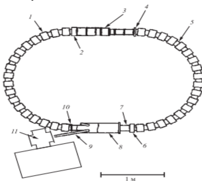
Рисунок 3 – Установка САТЕ. 1 – элемент фокусировки и поворота пучка; 2, 6 – ускоряющие зазоры; 3 – оптическая диагностика; 4, 10 – мониторы; 5 – вакуумная камера; 7 – малый соленоид; 8 – инфлатор; 9 – канал инъекции; 11 – электронная пушка и инжектор
