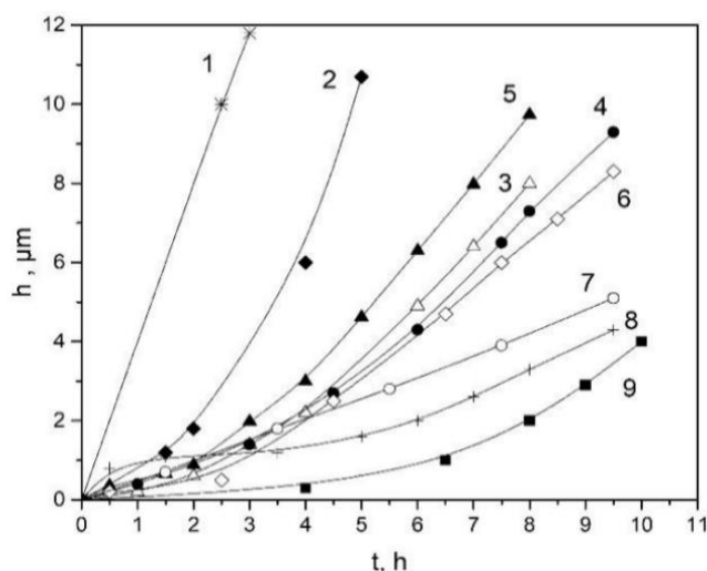
Рисунок 1 - Зависимость средней глубины эрозии ( h ) для титановых сплавов ( t ) 1 — ВТ1-0, 2 — ТЦ5, 3 — ВТ6, 4 — ВТ14, 5 — ОТ4, 6-19 — модифицированные ВТ6 и ВТ14 [2]
