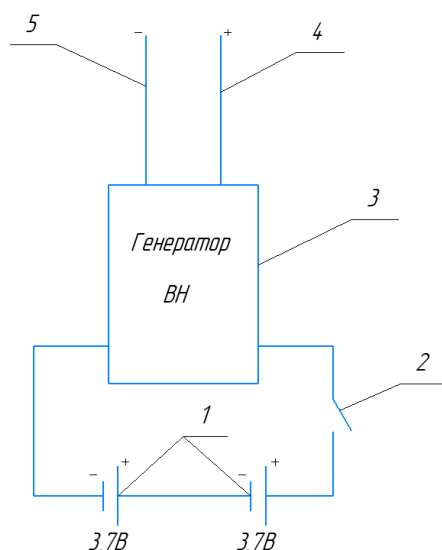
Рисунок 1 – Электрическая схема установки
