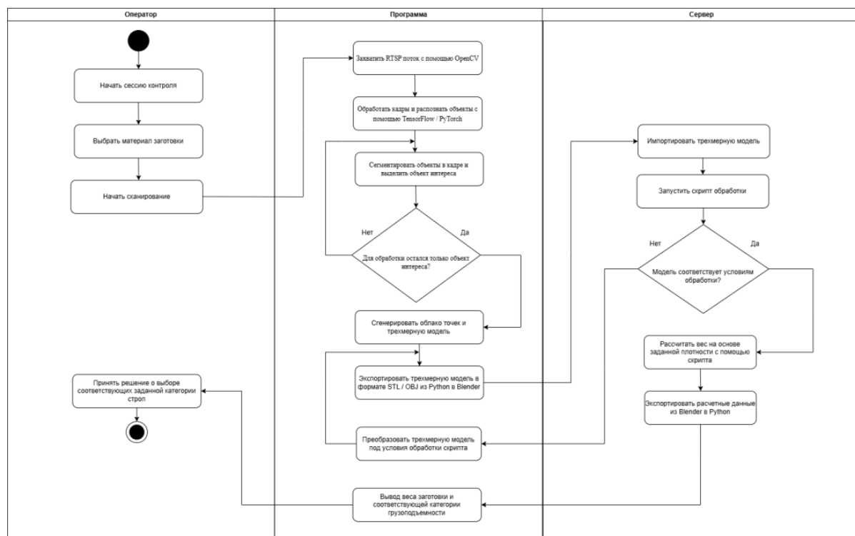
Рисунок 3 – Диаграмма деятельности
