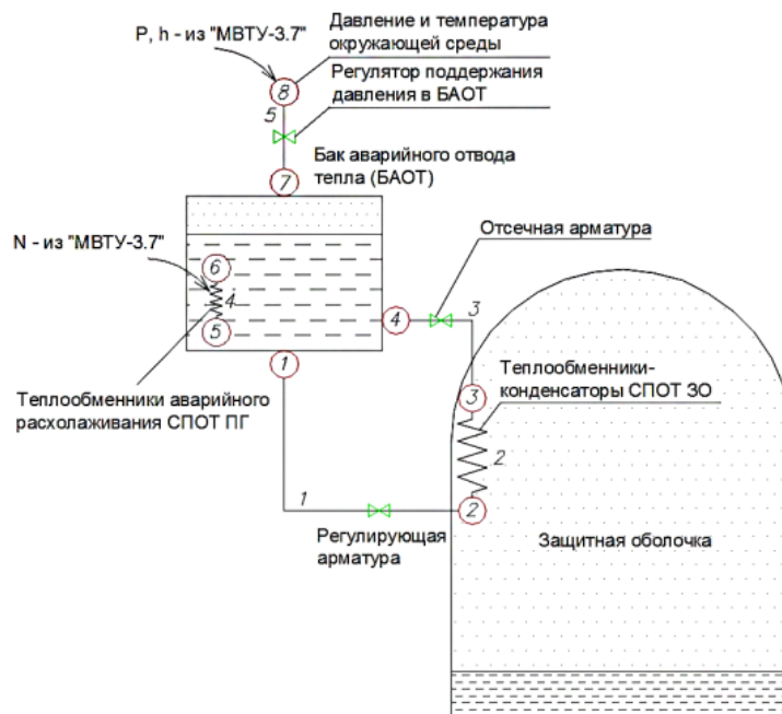
Рис 1. - Расчетная схема модели СПОТ 3О
