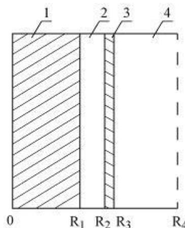
Рисунок 2 – Расчётная схема ТВЭЛ: 1 – слой топливных таблеток, 2 – гелиевый зазор, 3 – стенка ТВЭЛ, 4 – теплоноситель, R_1 – радиус поверхности столба таблеток, R_2 – внутренний радиус оболочки ТВЭЛ, R_3 – наружный радиус ТВЭЛ, R_4 – фиктивный радиус канала охлаждения [Design scheme of a fuel element: 1 – layer of fuel pellets, 2 – helium gap, 3 – wall of a fuel element, 4 – coolant, R_1 – radius of the surface of the column of pellets, R_2 – inner radius of the fuel element cladding, R_3 – outer radius of a fuel element, R_4 – fictitious radius of the cooling channel]
