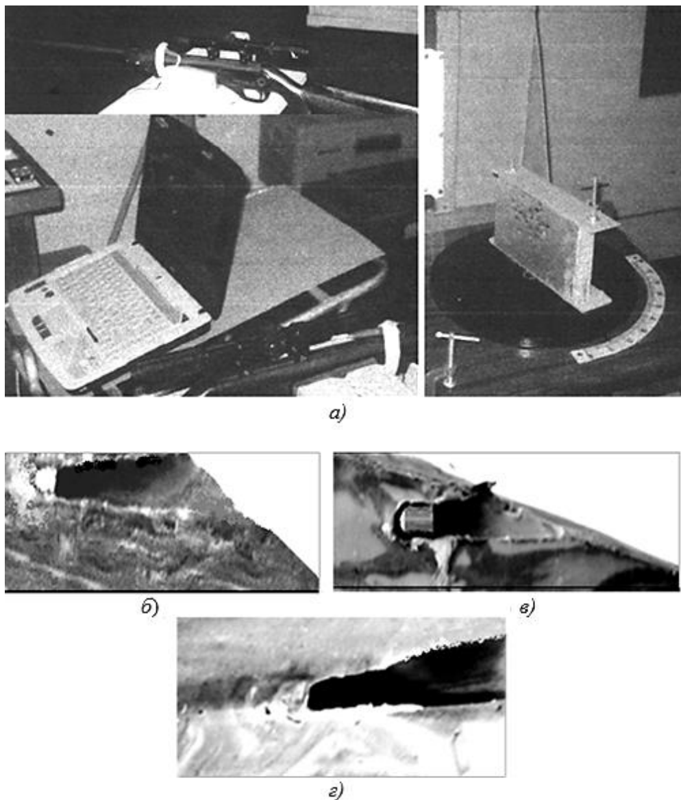
Рисунок 7 – Экспериментальные исследования процесса проникания ударников в вязкую среду: а – элементы экспериментальной установки; б – внедрение при \psi = 45^\circ ; в – внедрение при \psi = 70^\circ ; г – внедрение при \psi = 0^\circ [Experimental studies of the process of penetration of strikers into a viscous medium: a – elements of the experimental setup; b-introduction at \psi = 45^\circ ; c-introduction at \psi = 70^\circ ; d-introduction at \psi = 0^\circ ]
