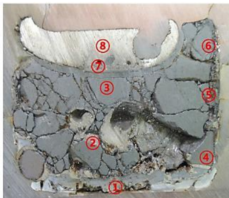
Рисунок 6 – Разрез образца кориума, полученного в процессе эксперимента, с указанием зон забора образцов [Cross-section of the corium sample obtained during the experiment, indicating the areas of sampling]
