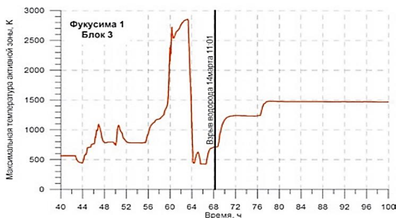
Рисунок 8 – Максимальная температура энергоблока 3 АЭС Фукусима Дайити в процессе аварии [Maximum temperature of Fukushima Daiichi Unit 3 during the accident] [21]
